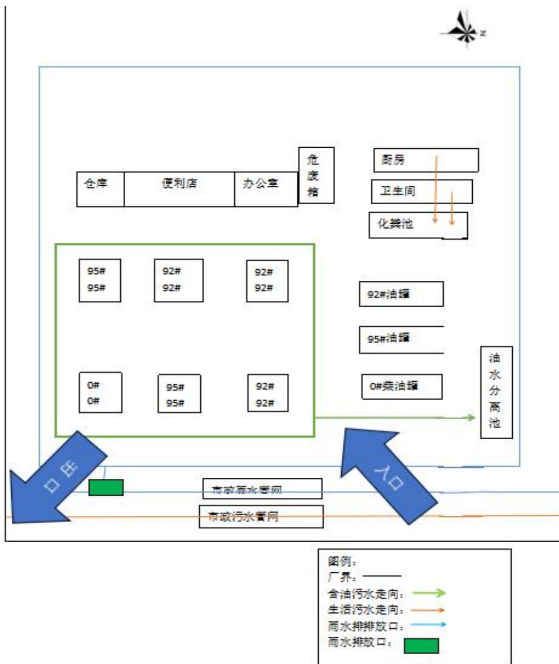
图2.3-1平面布置示意图
