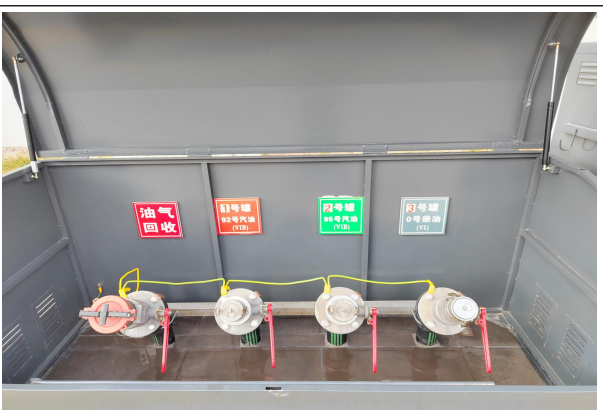
图 18 卸油口
