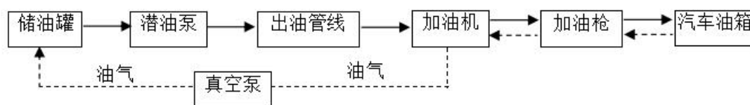
图2.4-1 汽油加油工艺流程图
