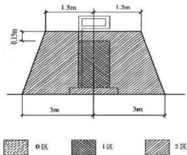
图 3.7-2 加油机防爆区域划分图
