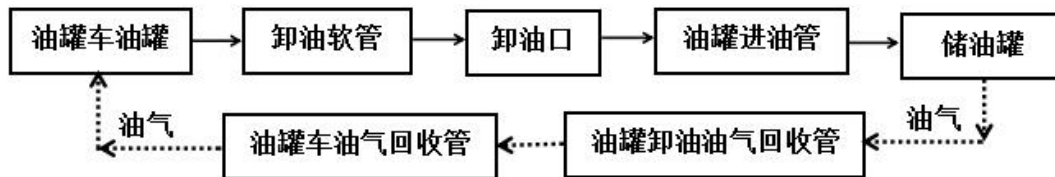
图2.4-4汽油卸油工艺流程框图
