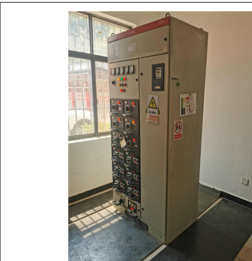
图 22、配电箱
