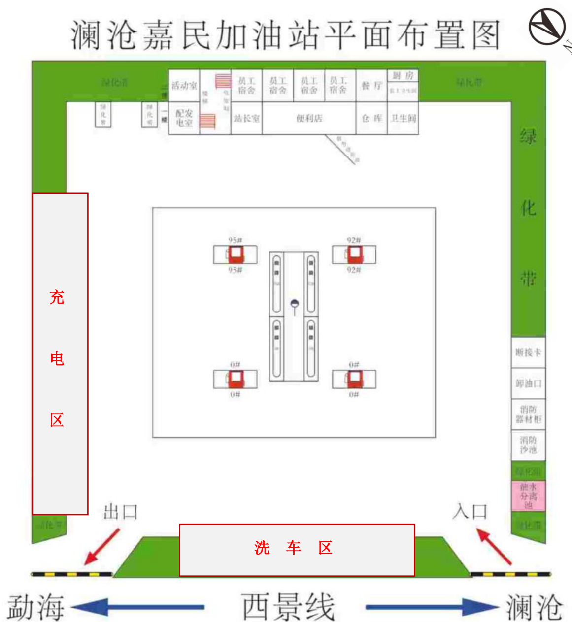
附件 14 加油站总平面布置图
