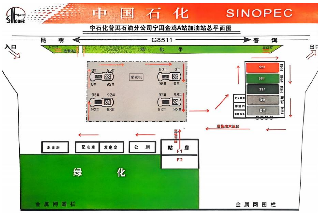
图2.3-1平面布置示意图
