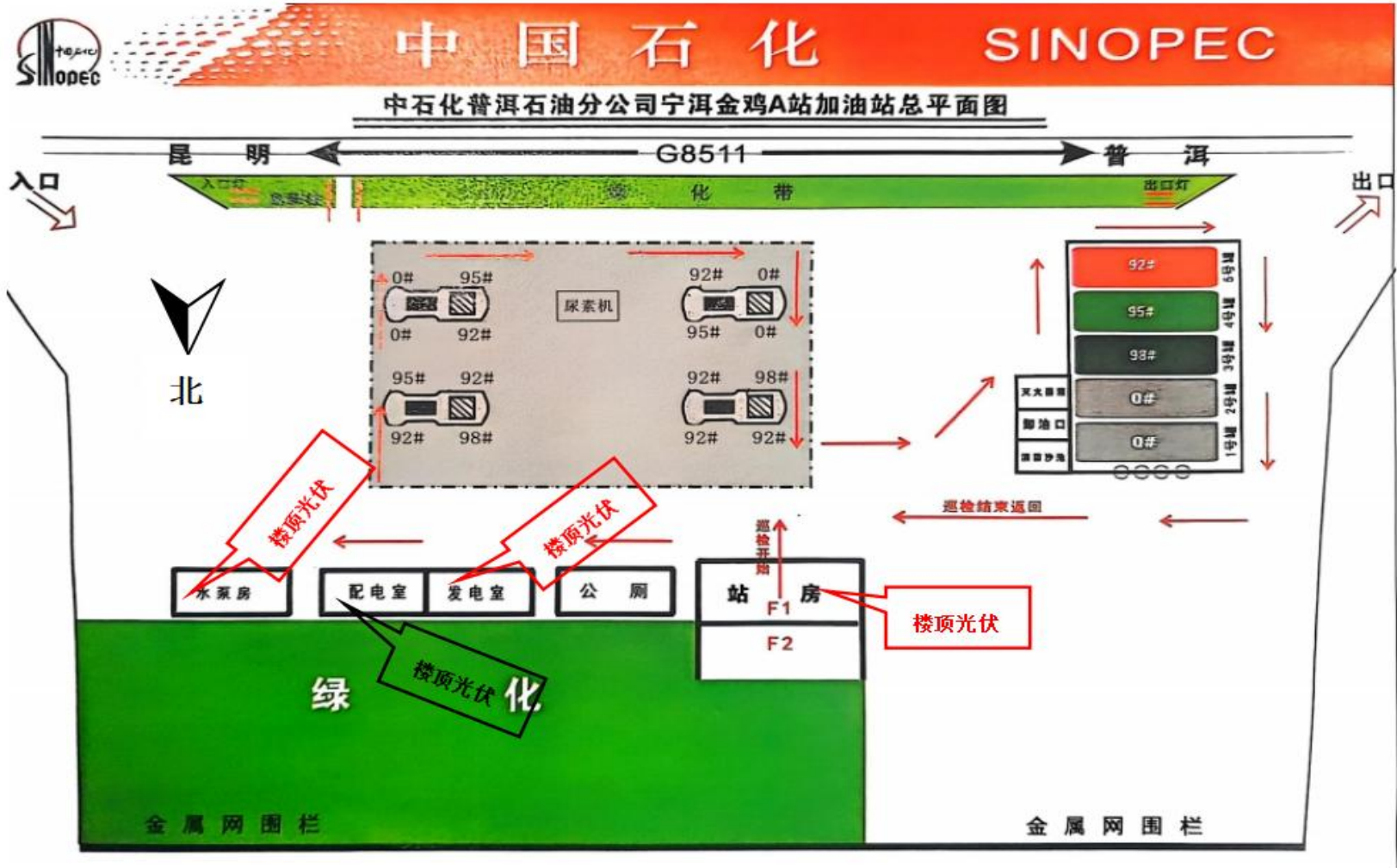
附件 16 加油站总平面布置图
