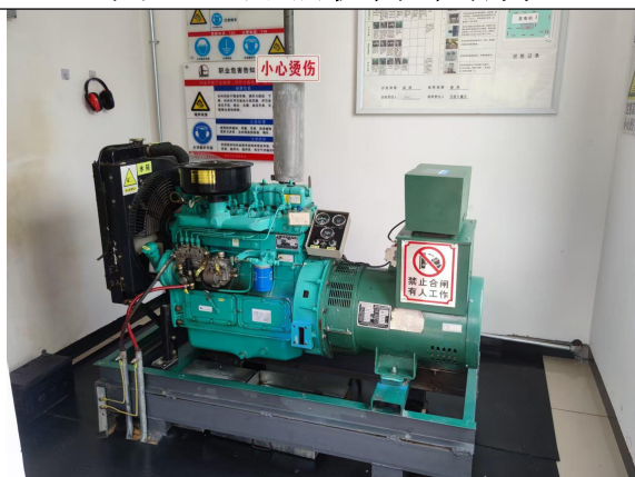
图 19 柴油发电机
