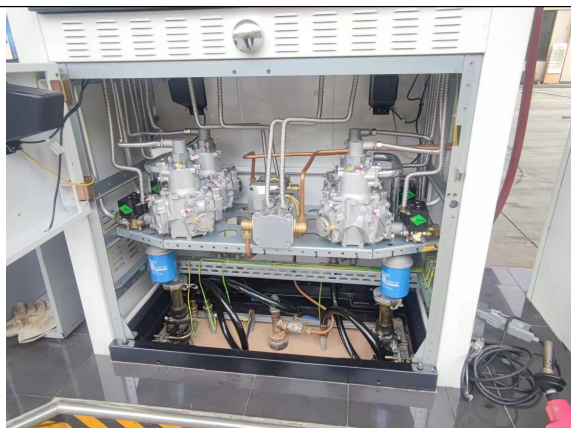
图 17 加油机内部结构
