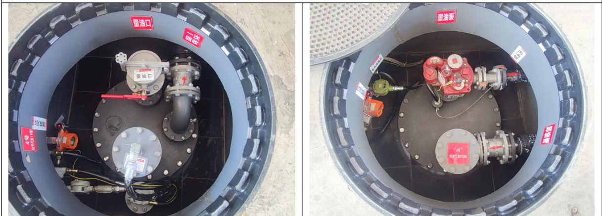
图 28 量油孔操作井
