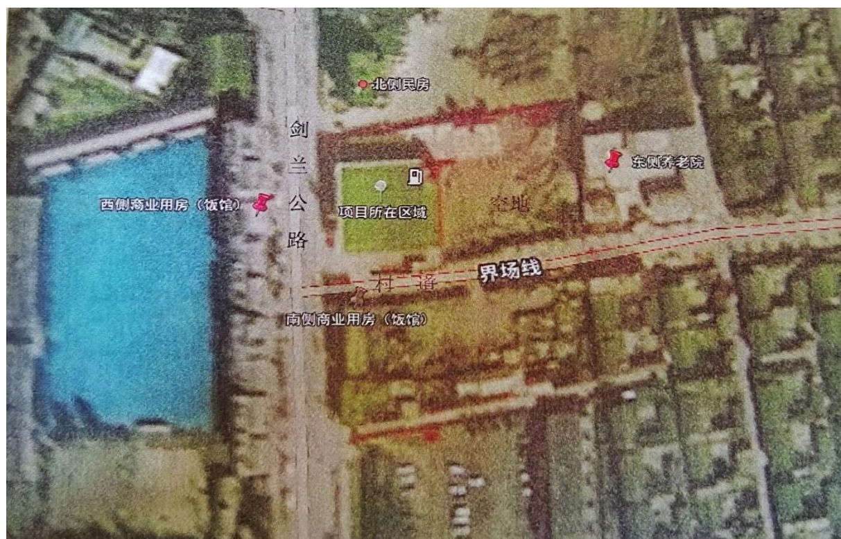
图 2-2 周边关系位置图
